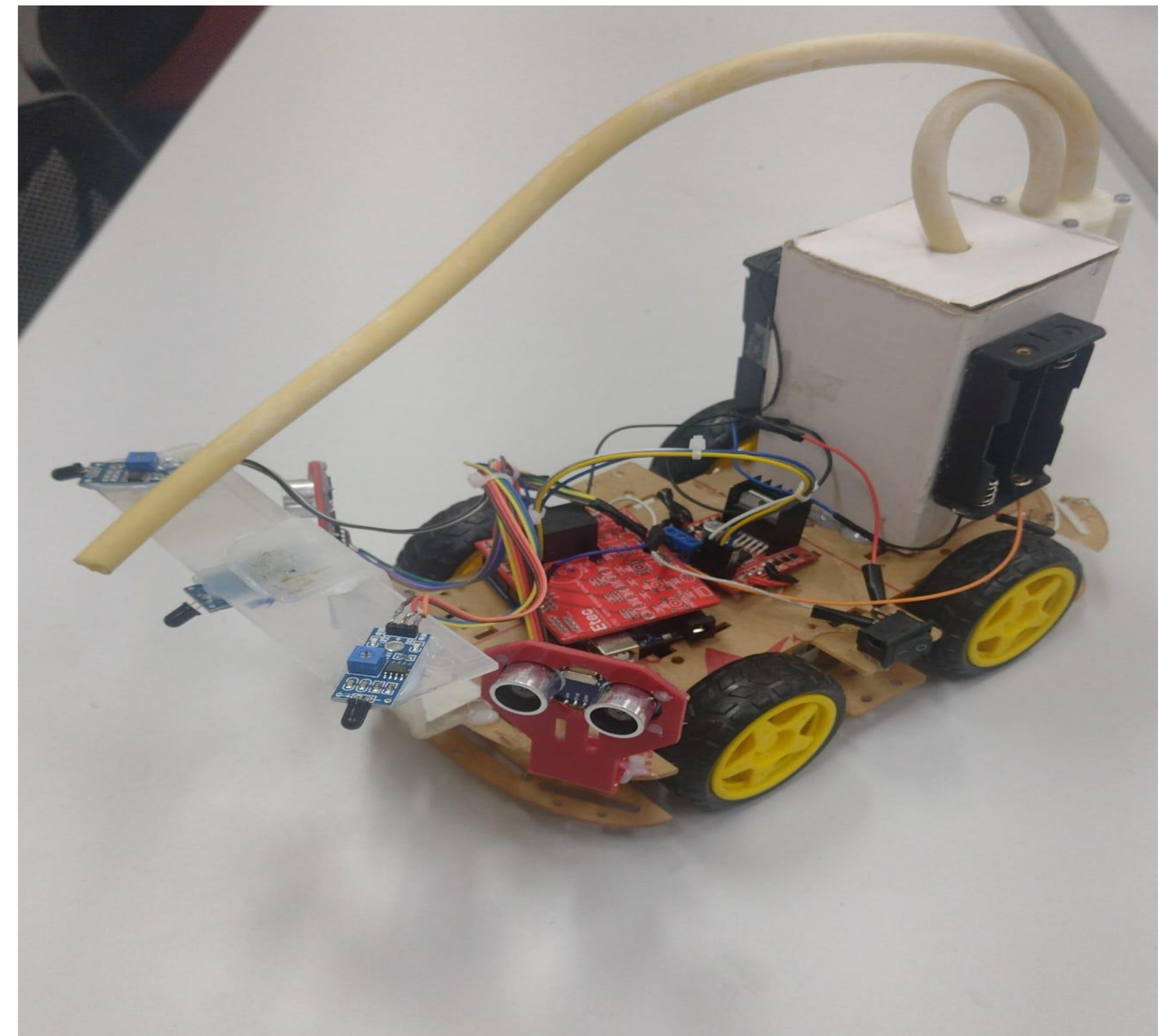
Fig. 01 – Robô de Combate a Incêndio
